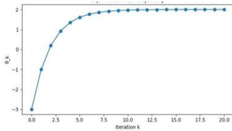
Figure 10. Parameter Trajectory
